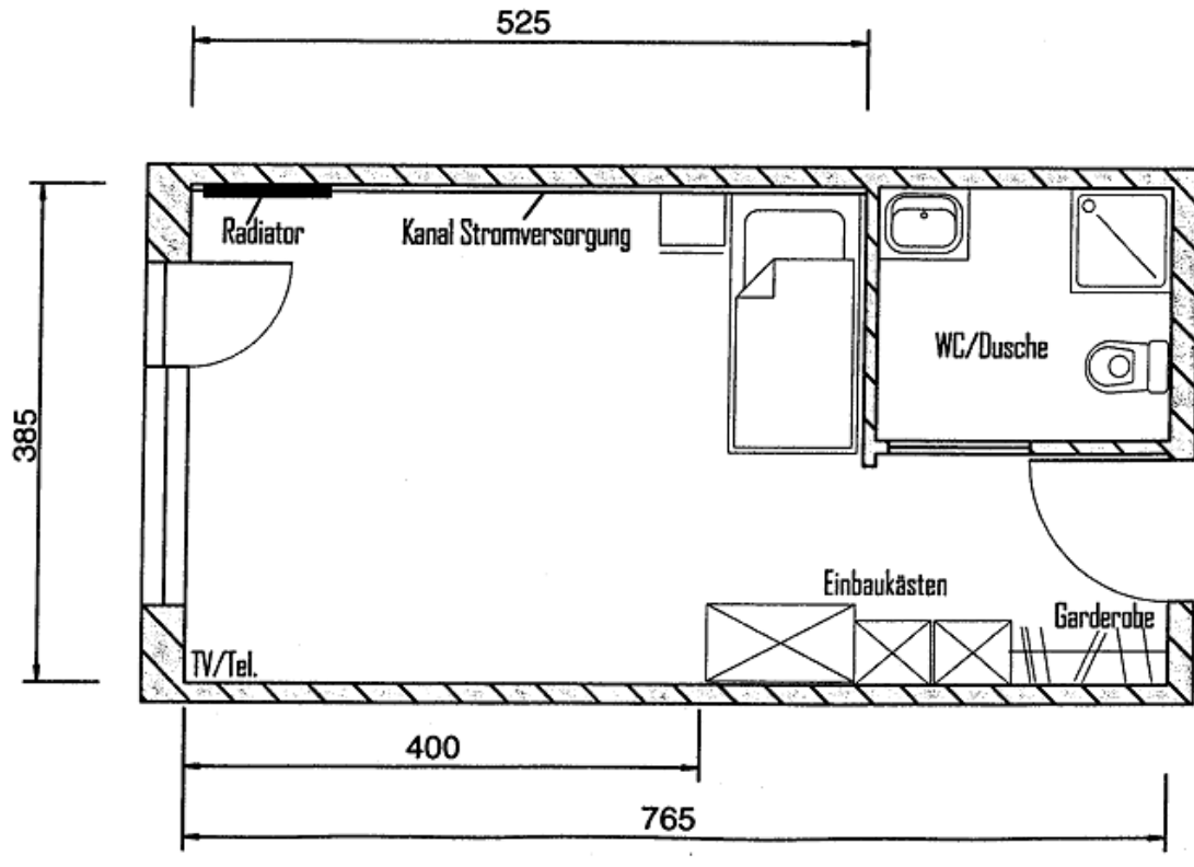
Zimmergrundriss (Duschzelle rechts)
